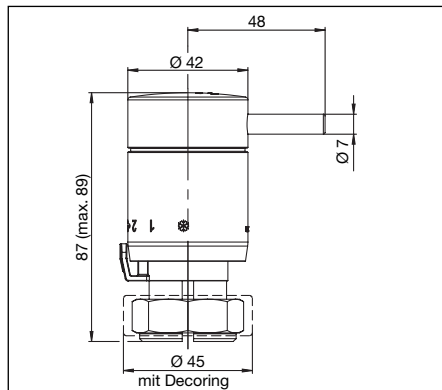
Abb. 4.1 Abmessungen
