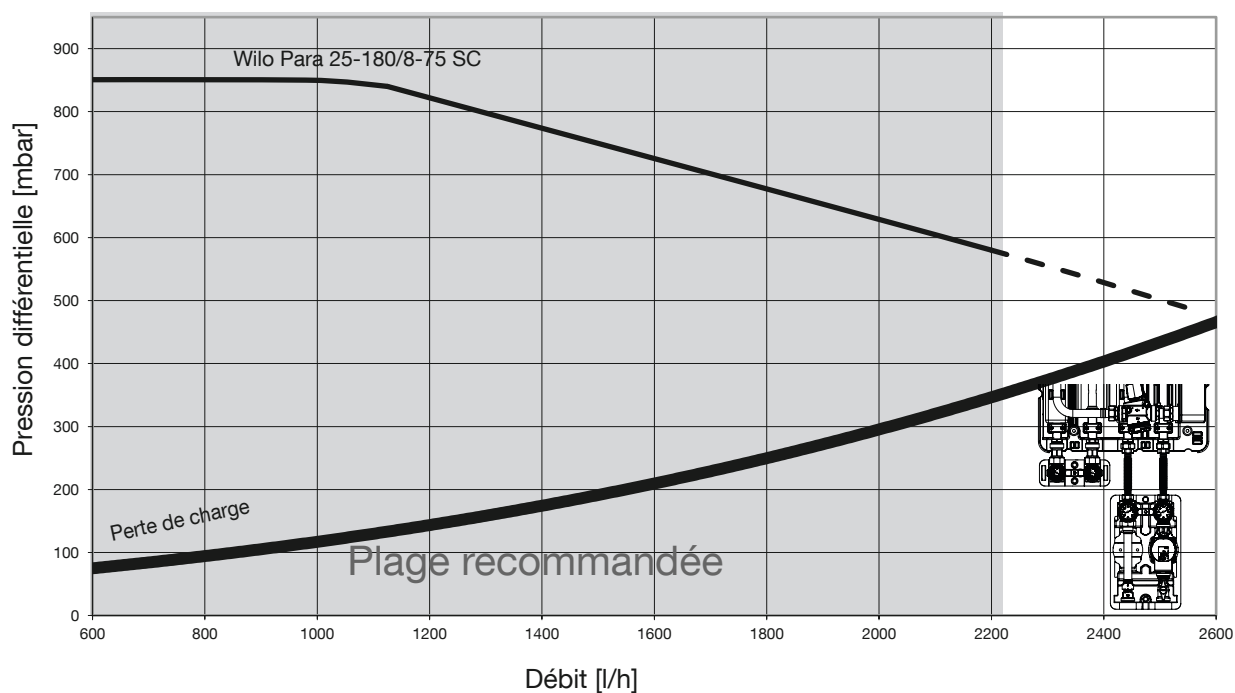
Fig. 5: Perte de charge circuit secondaire Regudis H-M
