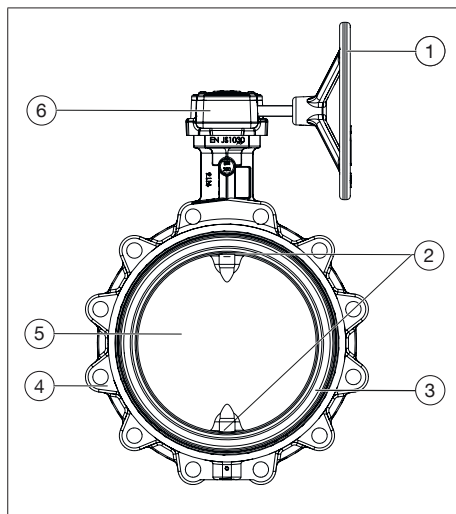
Fig. 1: Construction vanne papillon à réducteur à volant
