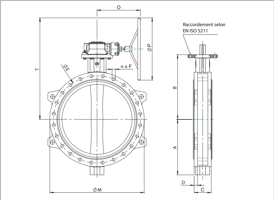
Fig. 6: Dimensions modèle à double bride DN 700 à DN 1400
