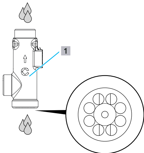
Abb. 23: Volumenstromsensor unter fließendem Wasser reinigen
