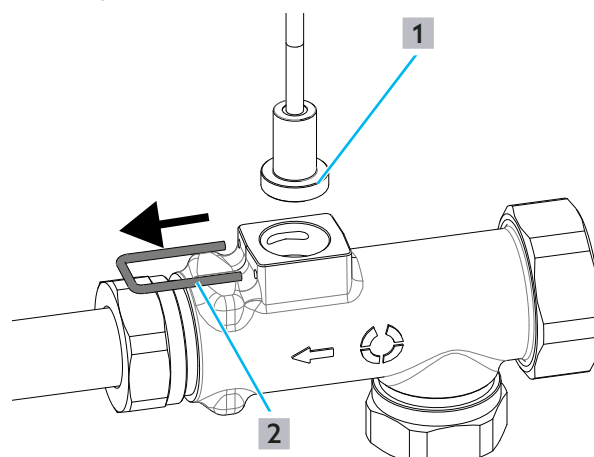
Abb. 21: Sicherungsklammer lösen
