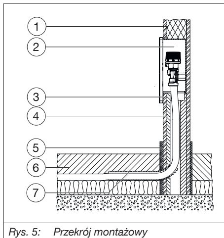
Rys. 5: Przekrój montażowy
