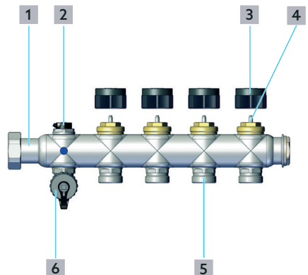
Fig. 2: Aufbau Rücklaufbalken
