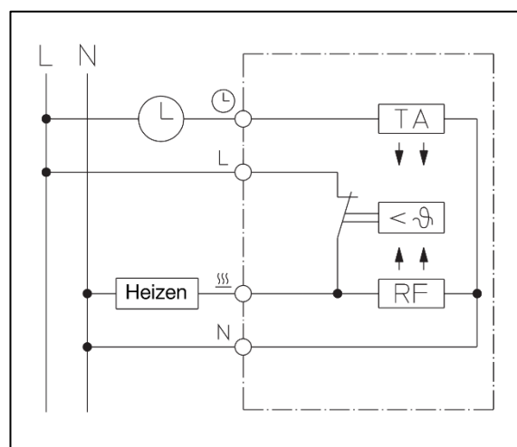
Schaltplan
