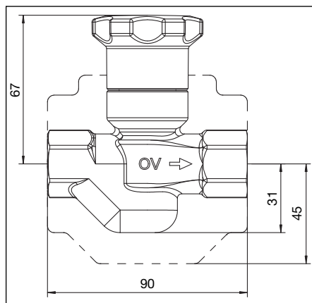
Fig. 4.2 Encombrements robinet avec coquilles d'isolation
