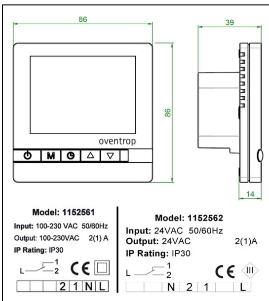
Abb. 4.1 Abmessungen
