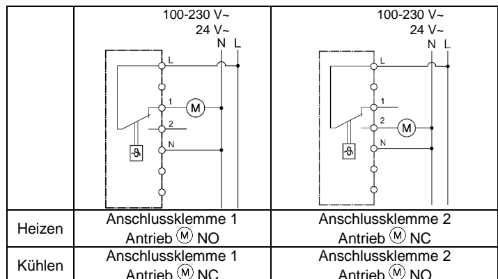
Abb. 6.2 Schaltplan Heizen/Kühlen
