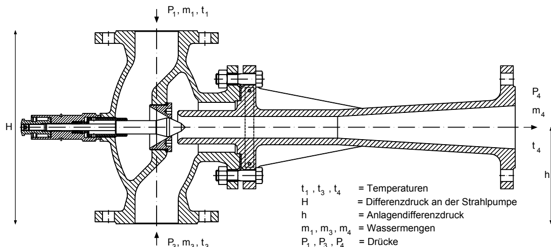
Bild 25: Geregelte Strahlpumpe
