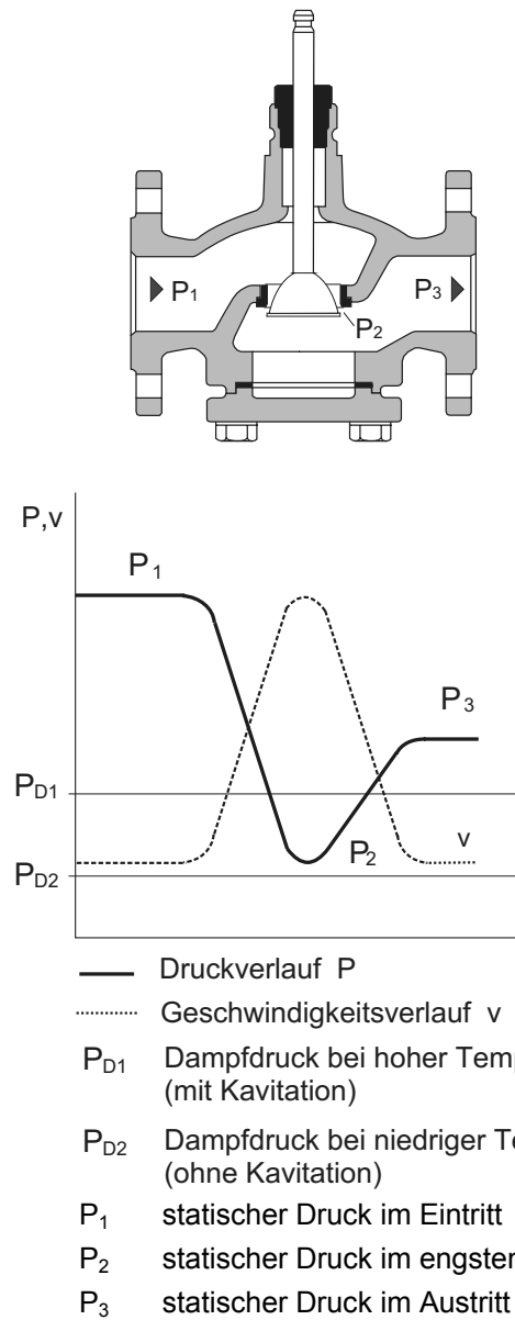
Bild 6: Druck-/Geschwindigkeitsverlauf im Regelventil
