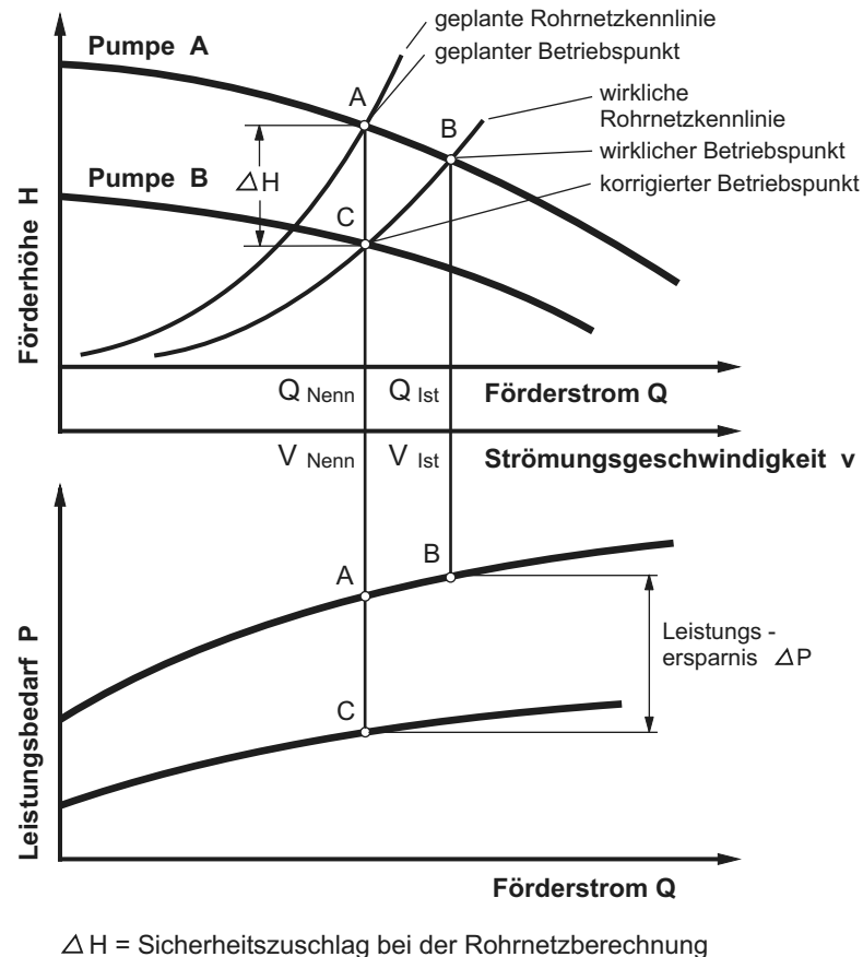
Bild 36: Leistungersparnis \Delta P
