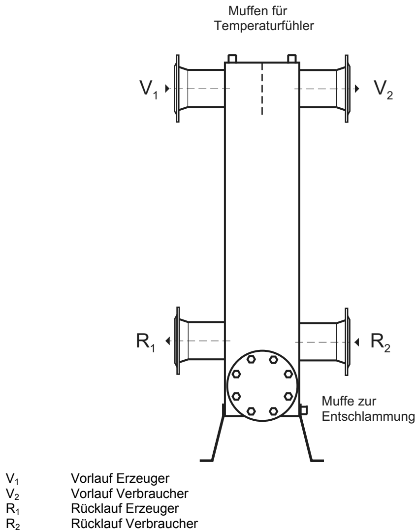
Bild 44: Hydraulische Weiche
