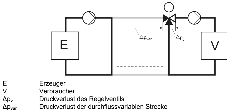
Bild 14: Beimischschaltung mit Entkopplung (Variante 3)
