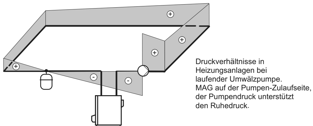
Bild 43: Druckverhältnisse in Heizungsanlagen
