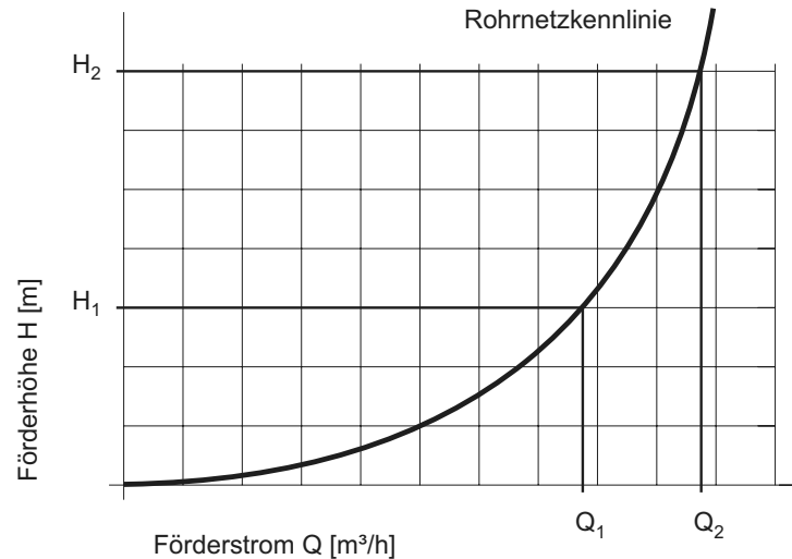
Bild 32: Rohrnetzkenlinie
