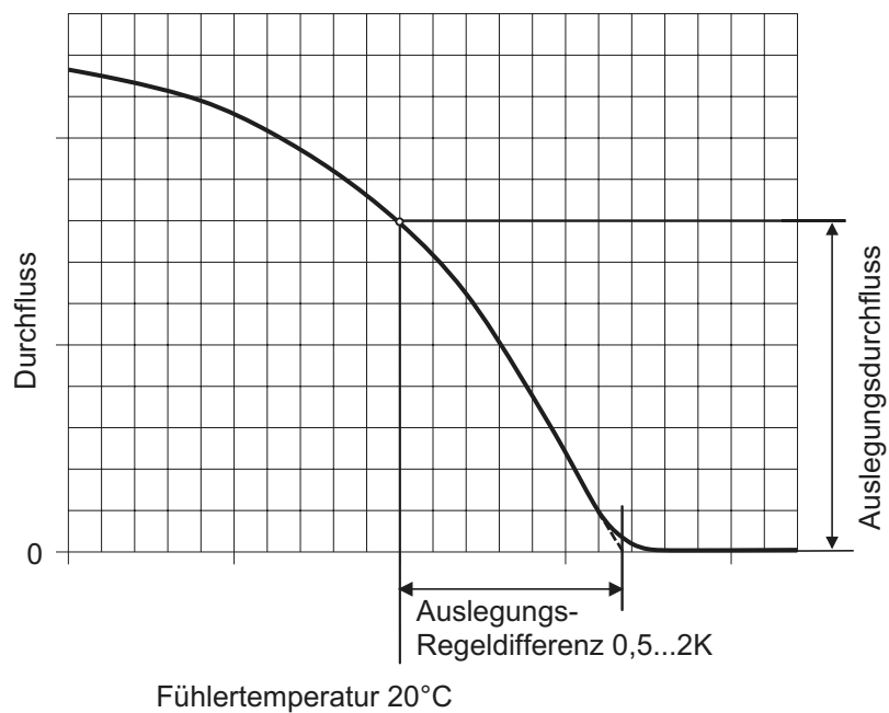
Bild 8: Auslegungs-Regeldifferenz bei Heizkörper-Thermostatventilen
