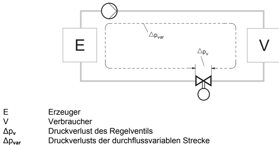
Bild 20: Drosselschaltung mit regelbarer Pumpe
