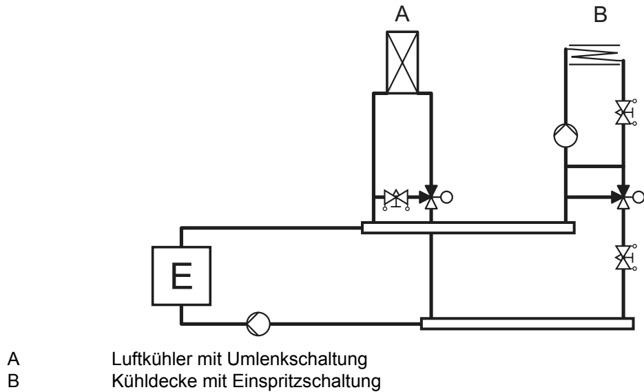
Bild 19: Kombination aus Umlenk- und Einspritzschaltung
