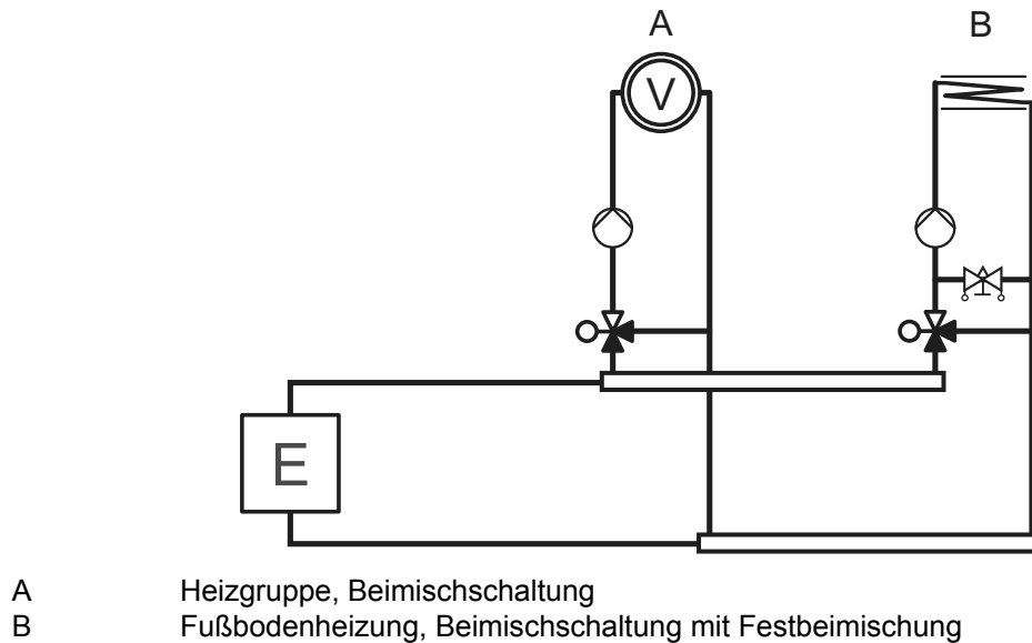
Bild 13: Kombination aus Variante 1 und Variante 2
