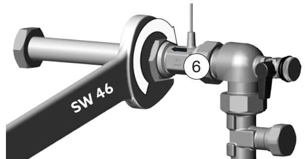
Abb. 5.16: Überwurfmutter Volumenstromsensor lösen
