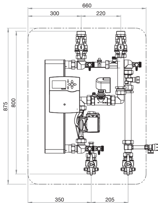
Abb. 3.8: Abmessungen „Regumaq X-70“ (Front)
