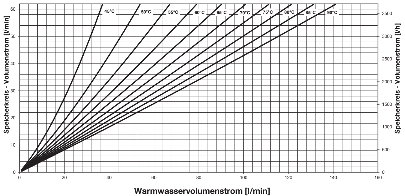
Rücklauftemperatur Speicherkreis bei unterschiedlichen Vorlauftemperaturen - Trinkwassererwärmung von 10 °C auf 45 °C -
