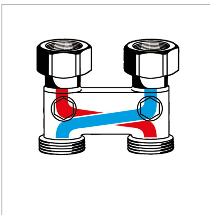
Racor de inversión con dispositivo de corte
