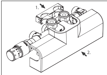
Abb. 12 Montage Design-Abdeckung
