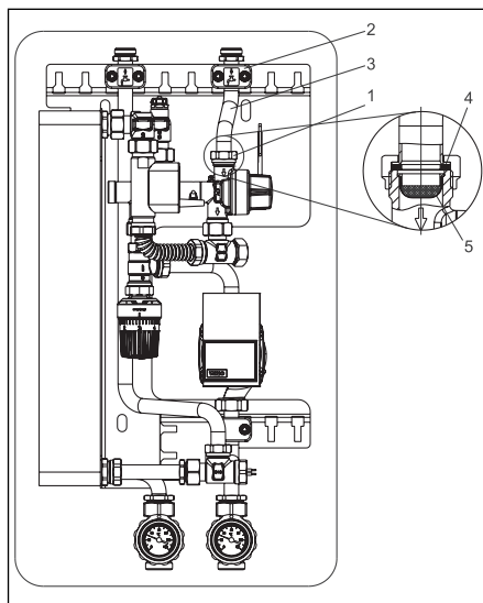
Fig. 5.1 Position de montage du tamis
