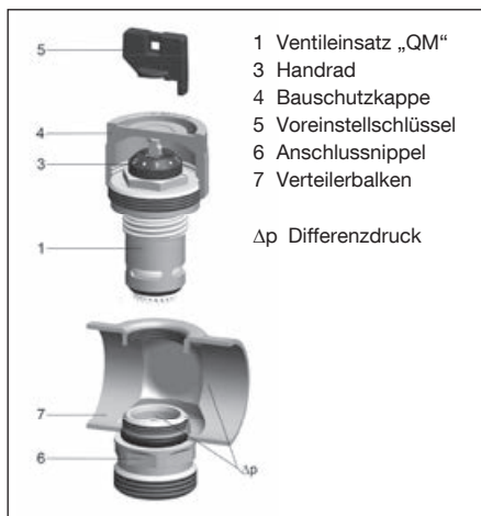
Abb. 5.1 Aufbau Ventileinsatz „QM“
