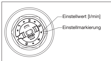
Abb. 7 Durchflusseinstellung
