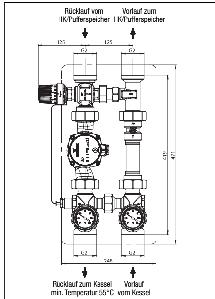
Abb. 4.6 „Regumat RTA-180“ DN32 mit Standardisolation Vorlauf auf der rechten Seite Kessel ist unterhalb der Station angeordnet
